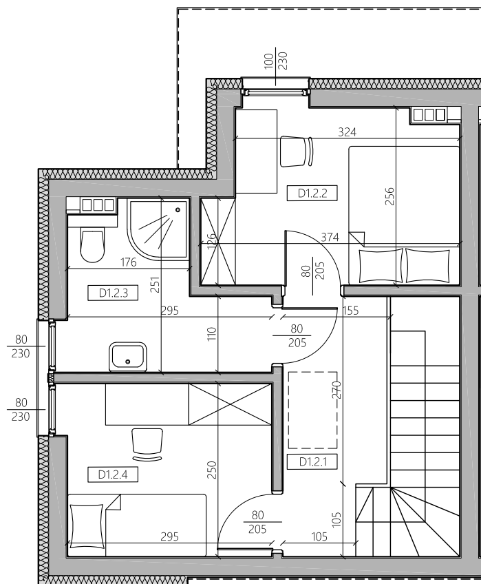
I PIĘTRO
